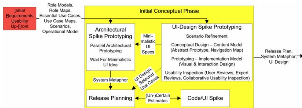
Abb.3: Initial Conceptual Phase des AUUSL
