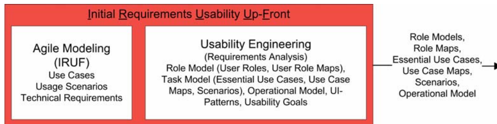
Abb.2: Phase „IRUUF“ (Initial Requirements Usability Up-Front) des AUCSL
